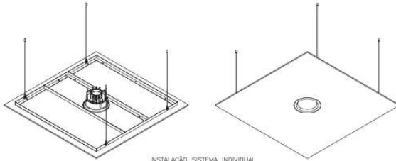
INSTALAÇÃO SISTEMA INDIVIDUAL COM TRAVA CABOS
