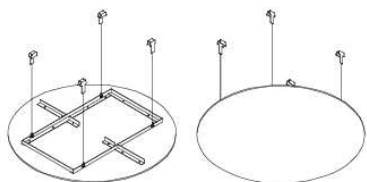
INSTALAÇÃO SISTEMA EM SÉRIE COM CALHA PERFILADA
