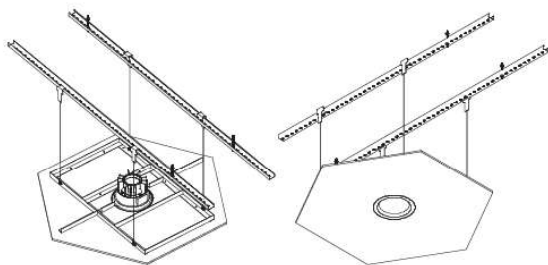
INSTALAÇÃO SISTEMA EM SÉRIE COM CALHA PERFILADA
