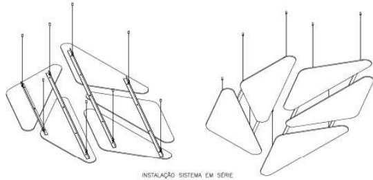
INSTALAÇÃO SISTEMA EM SÉRIE
