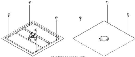
INSTALAÇÃO SISTEMA EM SÉRIE COM CALHA PERFILADA
