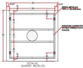
DETALHE QUADRO METÁLICO
