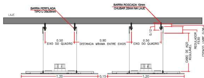
VISTA FRONTAL ESQUEMÁTICA
